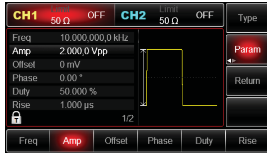
Figure 4- 26 Set rising edge
